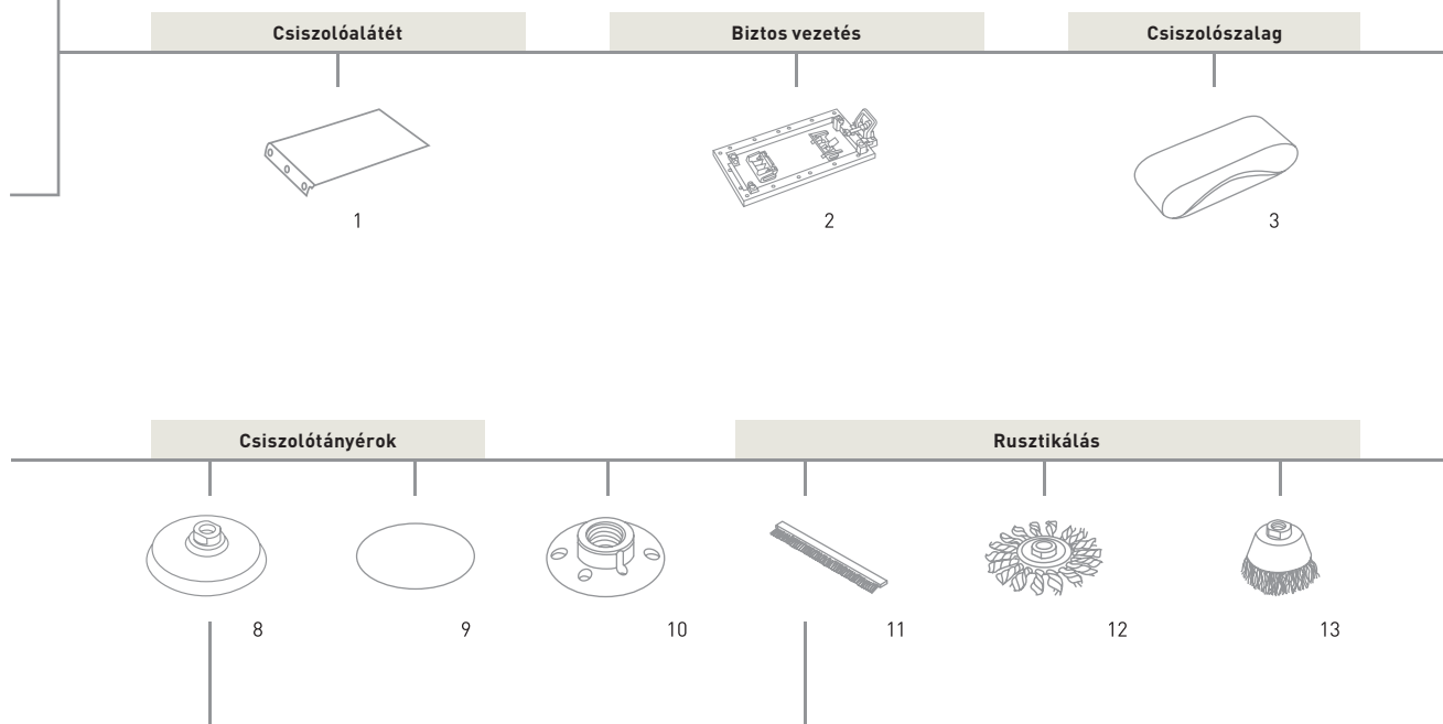
Szalagcsiszoló BS 105
