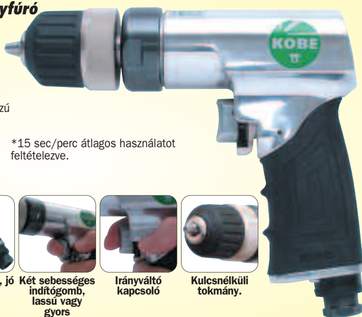
A kivezető csatlakozás a 360°-ban állítható.
